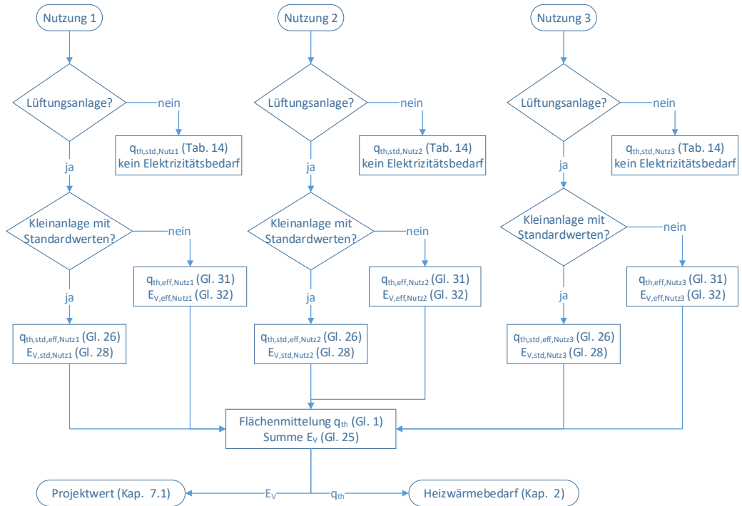
Abb. 5 Flussdiagramm Berechnung wirksame Aussenluftvolumenströme und Elektrizitätsbedarf.
